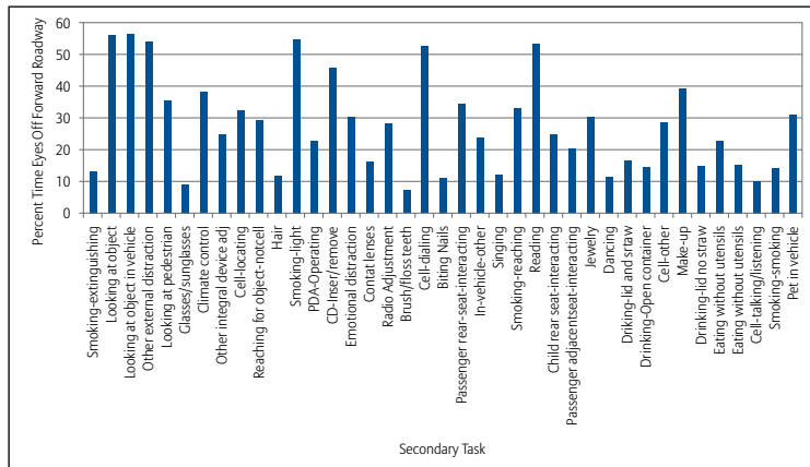
Bild 23: Wohin schaut der Fahrer, wenn er fährt? Die 100Car-Naturalistic-Driving-Study der US NHTSA (100Car-Study, 2010)
